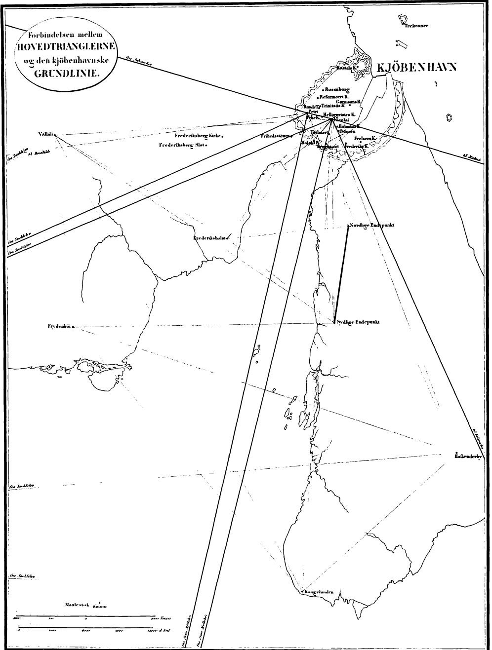
Reproduktion af Tab. III i C. C. G. Andræ: Den danske Gradmaaling, Bind 1 , der viser Forbindelsen mellem Hovedtrianglerne og den københavnske Grundlinie.
