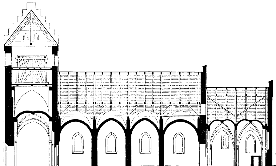
SØBORG KIRKE LÆNGDESNIET
