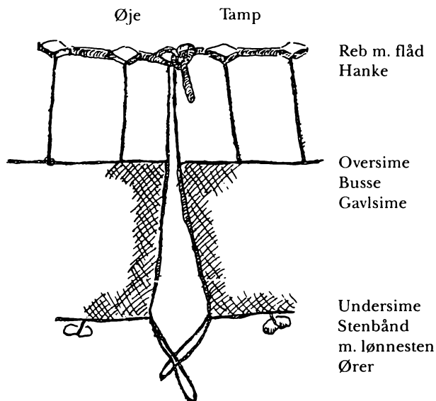
Detail af sammenbinding. (Hankegarn tegnet efter anvisning af L.P. Petersen, Reersø). Skitse af Holger Rasmussen.
