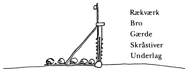
Tværsnit gennem et fang.
