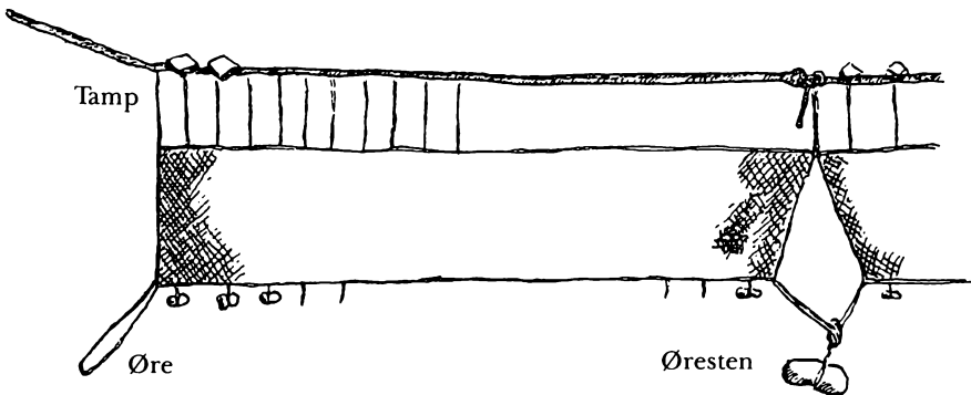
Reersø. Hankegarn. Man ser et helt garn og forbindelsen til det næste. Skitse af Holger Rasmussen.
