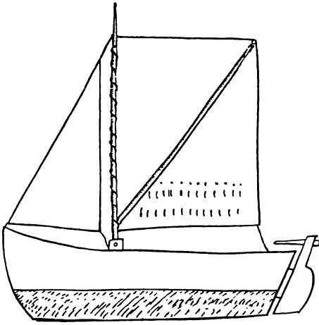
Reersø. Spejlgattet bæltsbåd med sprydejæl og dæk til masten. Set fra siden og bagfra. Skitser af Holger Rasmussen.
