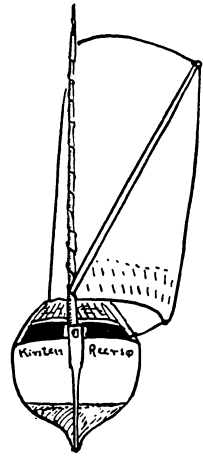
Reersø. Spejlgattet bæltsbåd med sprydejæl og dæk til masten. Set fra siden og bagfra. Skitser af Holger Rasmussen.
