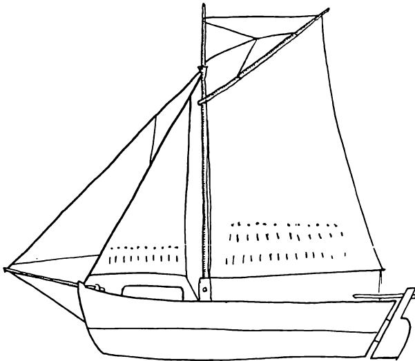
Reersø. Rundgattet bæltsbåd med gaffelsejl. (Tegnet efter skitser af bådebygger L. P. Larsen, Reersø). Skitse af Holger Rasmussen.
