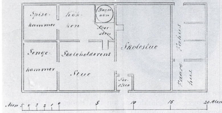
Plan over rytterskole fra 1739, udarbejdet af tømrer Bielenberg i Holbæk. Samme model blev benyttet til skolen i Skellebjerg.
