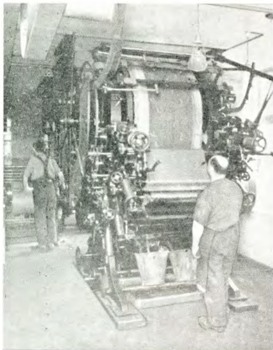
Tapettrykkemaskine med 8 Farver.
