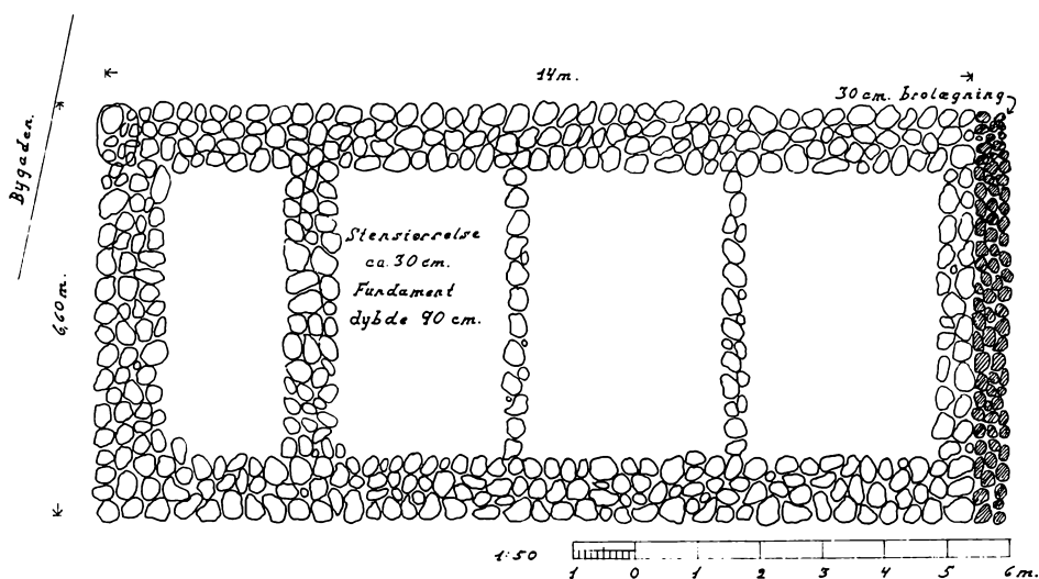
Fundament udgravet 1964
