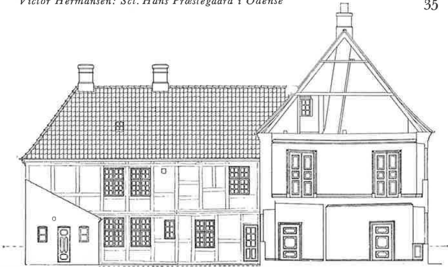
Sct. Hans Præstegaard. Tværsnit gennem Hovedbygningen og Vestside af Nørregade-Fløjen
