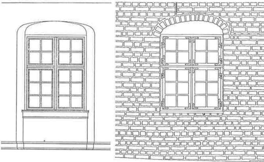
Sct. Hans Præstegaard. Vindu (inde fra) og Murværk fra 1636 1 : 50. Maalt af Jørgen Hvenegaard Lassen 1941
