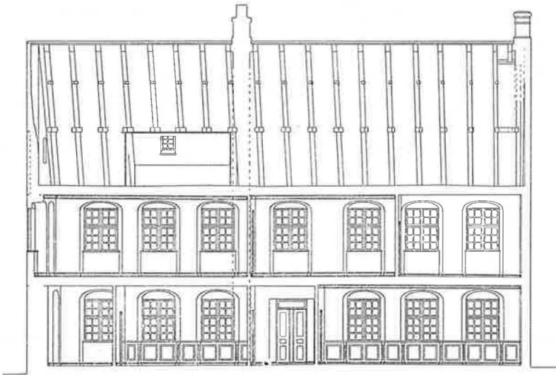
Sct. Hans Præstegaard. Længdesnit af Hovedbygningen, set mod Syd 1 : 200. Maalt af N. Jacobsen 1905
