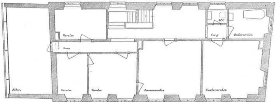
Sct. Hans Præstegaard. Plan af Førstesal 1 : 200. Maalt af Jørgen Hvenegaard Lassen 1941
