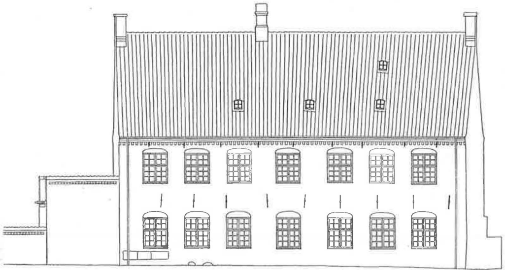
Sct. Hans Præstegaard. Sydside, mod Kirkepladsen 1 : 200. Maalt af Jørgen Stærmose 1941
