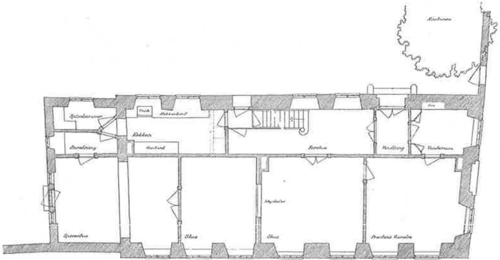
Sct. Hans Præstegaard. Plan af Stueetagen 1 : 200. Maalt af Jørgen Stærmose 1941
