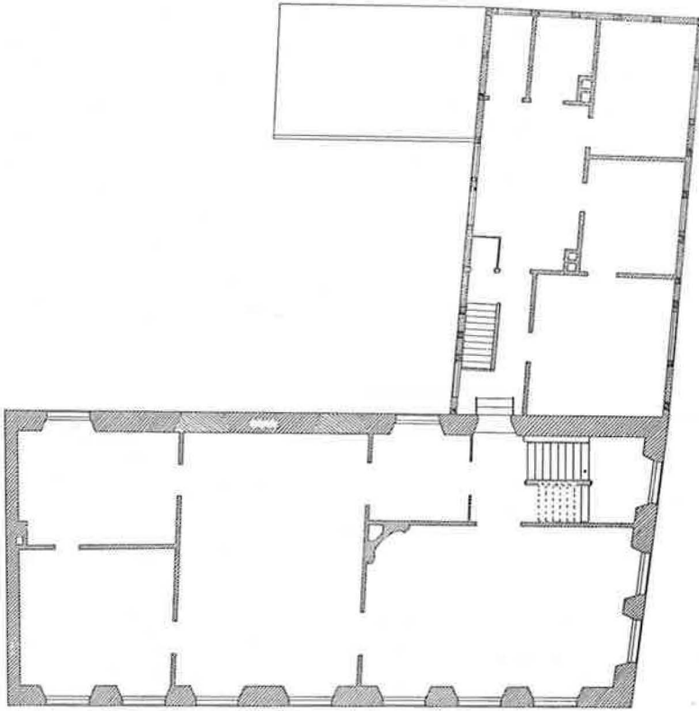
Sct. Hans Præstegaard. Plan af Førstesal 1 : 200. Maalt af N. Jacobsen 1905
