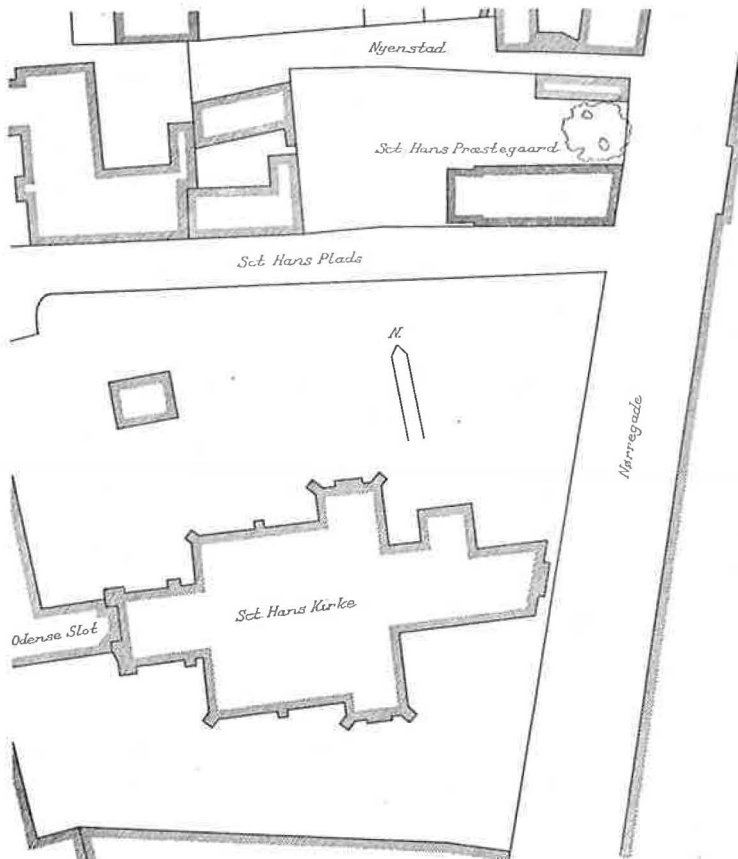
Sct. Hans Kirke og Præstegaard. Situationsplan 1 : 1000. Maalt af Jørgen Hvenegaard Lassen 1941
