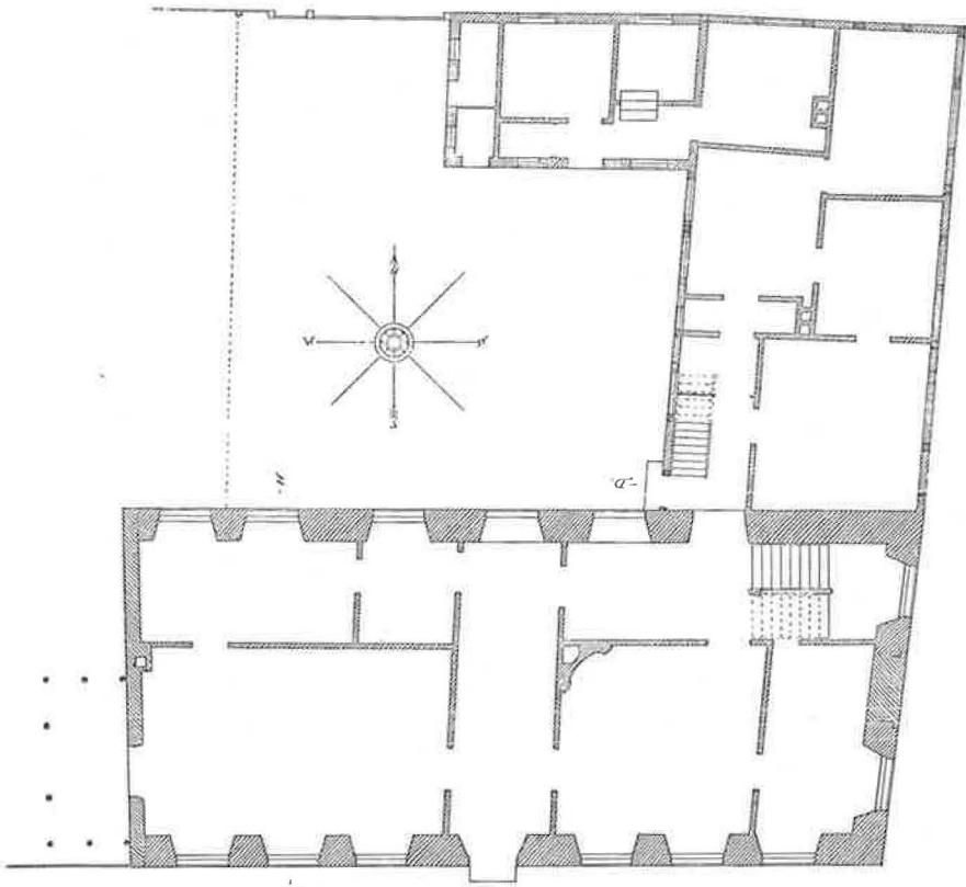
Sct. Hans Præstegaard. Plan af Stueetagen 1 : 200. Maalt af N. Jacobsen 1905
