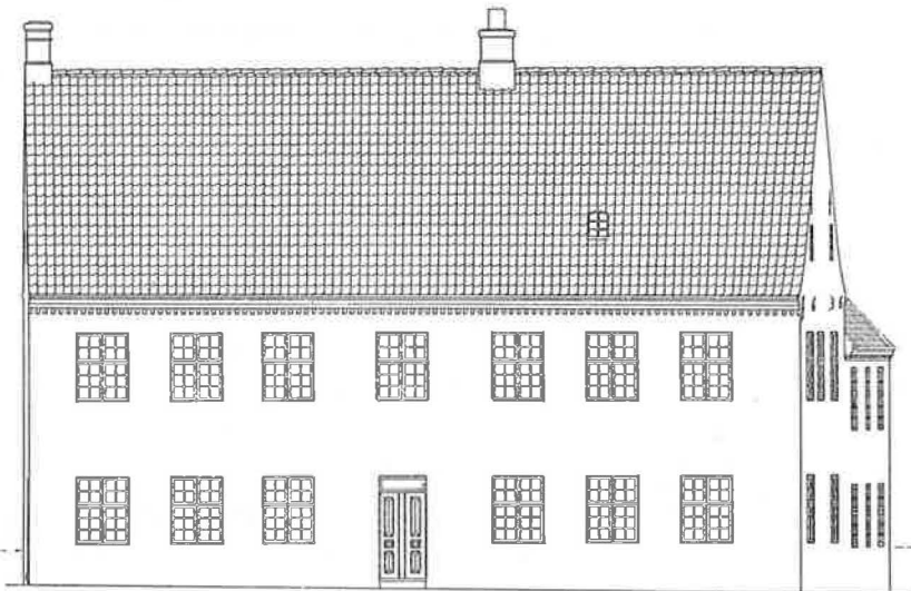
Sct. Hans Præstegaard. Sydside, mod Kirkepladsen 1 : 200. Maalt af N. Jacobsen 1905
