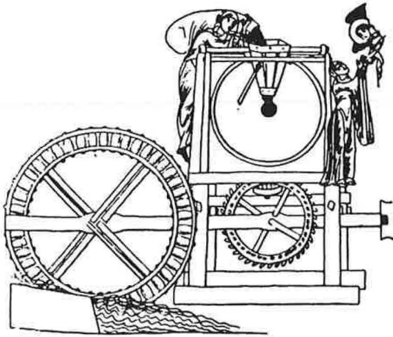
Fig. 3. Vandmølle med lodretstillet underfaldshjul. Kværnen og hjuludvekslingen er vist skråt fra oven. Tegning af Herrad von Landspergs »Hortus Deliciarum«, o. 1170 (ef. H. Gleisberg 1956).
