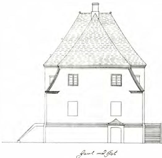
Constantinsborg. Østgavlen efter tegning af C. Steinbrenner fra 1867.
