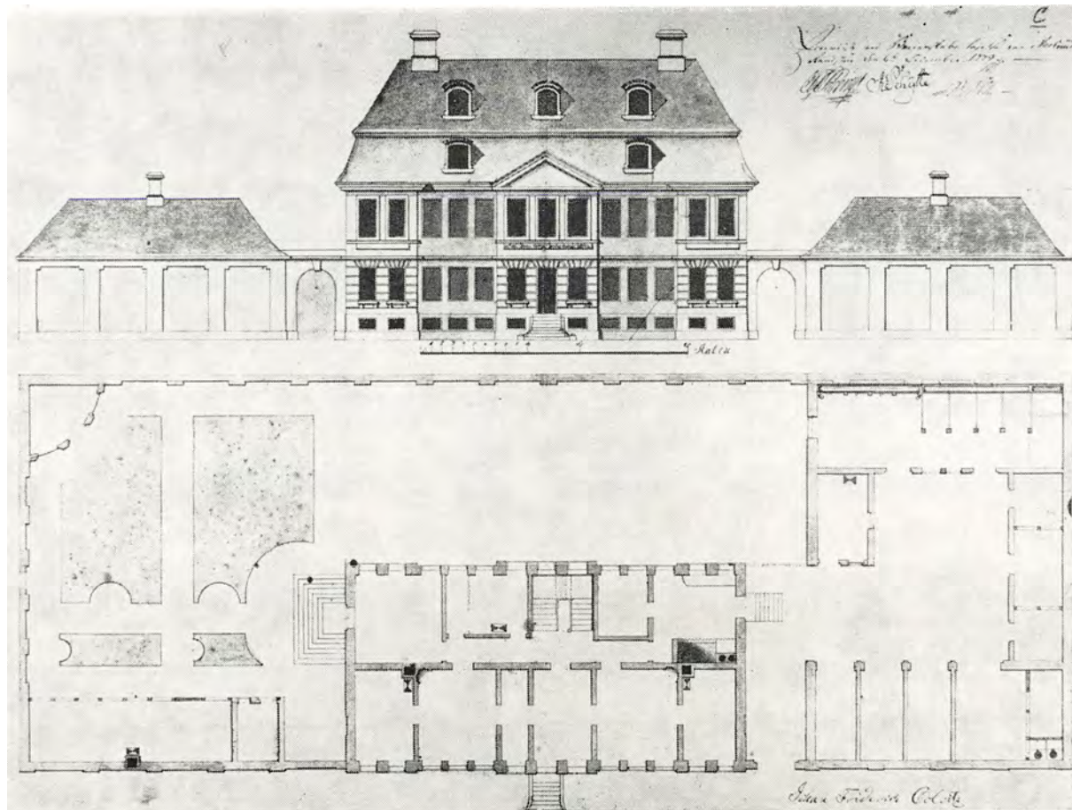
Mestertegning af J. F. Colwitz fra 1780 i »Den gamle By«.
