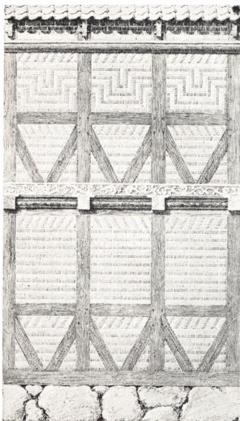
RAADMAND CHR. THOMSENS HUS; tre Fag Bindingsværk og mønstermurede Tavler, efter Rekonstruktion af Prof. Mejborg; Tegn. i Nationalmus.
