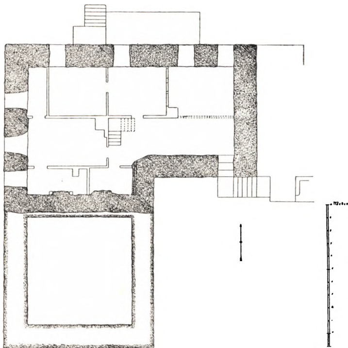
STENHUS OG TAARN, Opmaaling af Kældrene under Slottet ved la Cours Undersøgelse 1904 (Nationalmuseet). Det skraverede er Stenhusets Mure med den lille Tilbygning, der forbandt det med Taarnet, hvis kvadratiske Grundplan er antydnet paa Tegningen.
