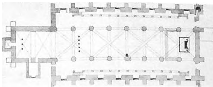
Thuras Grundplan af Maribo Kirke 1736.
