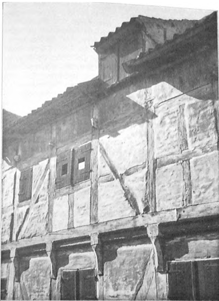
Badstuestræde, Theisens »Strædeloft«. Typisk nakskovsk Pakhusbindingsværk fra det 18. Aarhundrede: under det fremspringende Tagskæg uden Tagrende ses »Styrterummet«; de øverste Bjælkehoveder er gennemstukne; store Skraastivere; Stokværks»udkrøgning«(fremspring); rygskaarne Knægte under de nederste Bjælkehoveder. *
