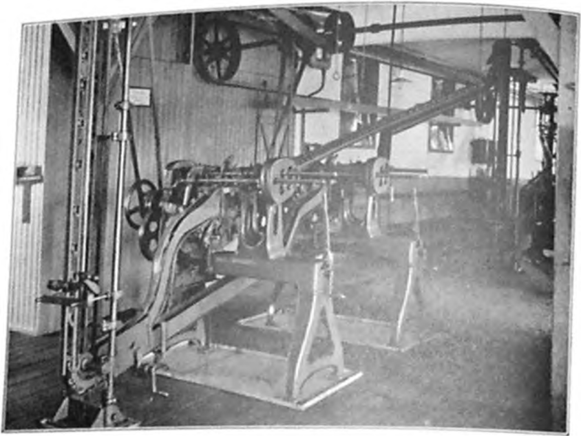
Kondenseringsfabriken. Bertlemaskine paa Daasefabrikken. Fra Blikpladen lægges i Rullesaksen og til de fyldte Daaser triller ud paa Pakkerskernes Borde, foregaar alt automatisk.
