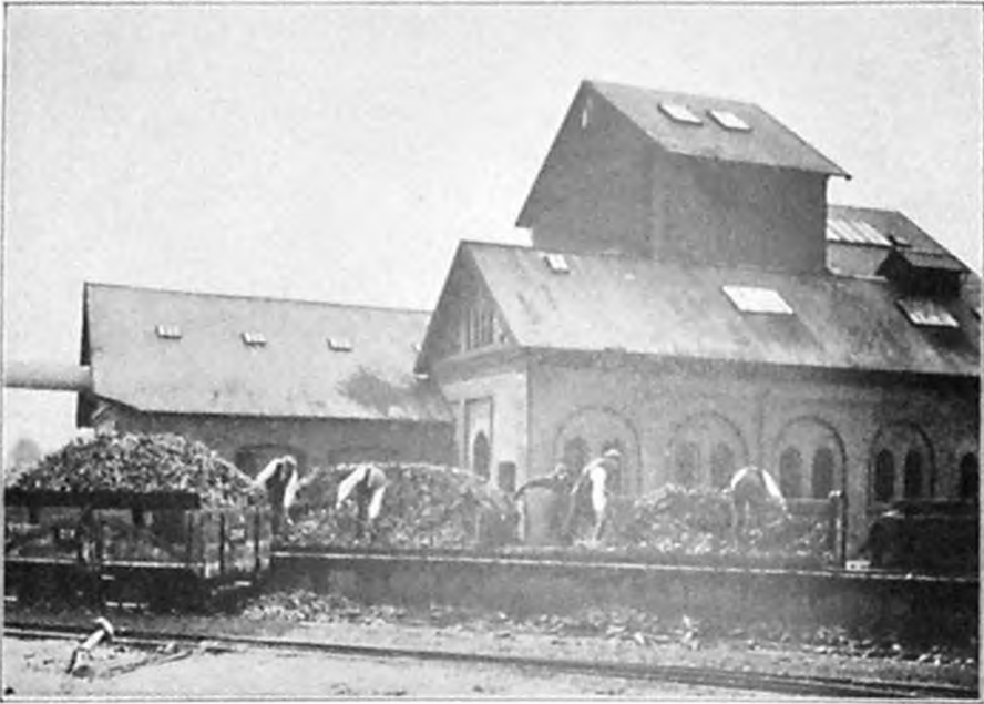
Sukkerfabriken. Fra »Sporvognene« læsses Roerne af i »Svømmerenden«, hvori de sejler ind i Saftstationen.
