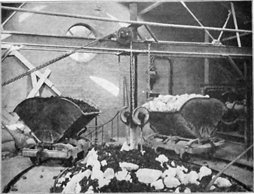
Roesaften renses med brændt Kalk. Her er vi paa Kalkbrænderiets Loft, hvor Kalk og Cinders styrtes ned i Ovnens Ildsvælg.
