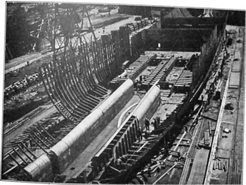
Værftets Nybygning Nr. 60, fot. d. 24. Maj 1934. Baaden søsattes d. 11. August under Navnet »Jutlandia« og afleveredes d. 11. November 1934 til »Ø. K.«
