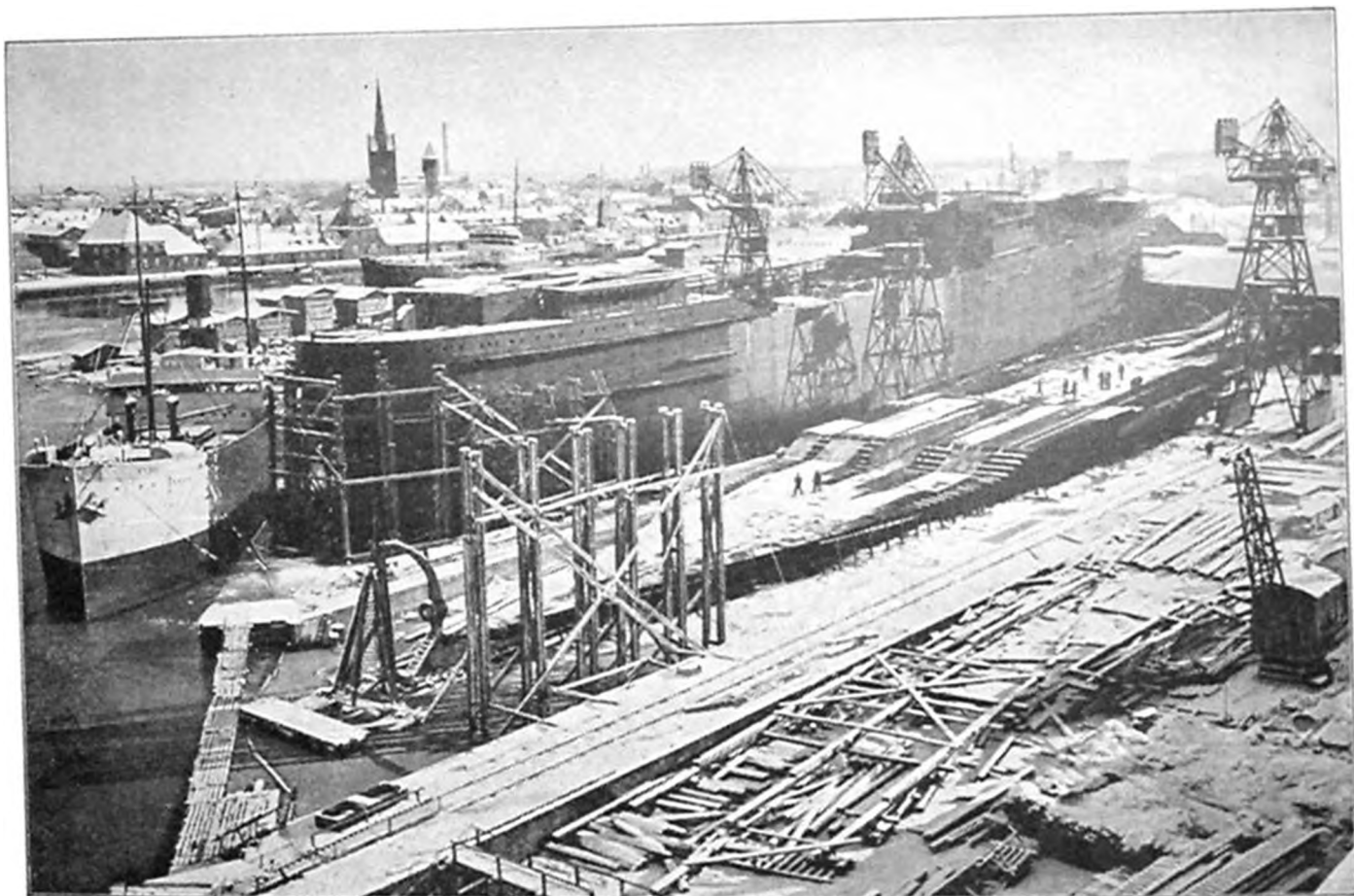
Nakskov Skibsværft 6. Febr. 1935. Det store Skibsskrog er en Nybygning, 12,750 Ts, til »The Texas Company», T. M. S. »Brasil»; foran dette Bunden og Agterstævnen til O. K.'s M. S. »Canada». Ved Beddingekajen I. Lauritzen's S. S. »Else», ved Havnekajen O. K.'s »Mexico».
