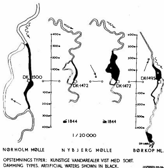
Plan 1/20 000 af Nørholm, Nybjerg og Børkop Møller. Opstemningsarealerne er vist med sort.
