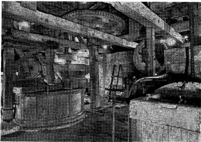
Interiør fra Nørholm Møllens kværnloft, hjul 1. Til venstre i billedet ses stenkranen, hvormed man vender overstenen, naar kværnen skal billes.
