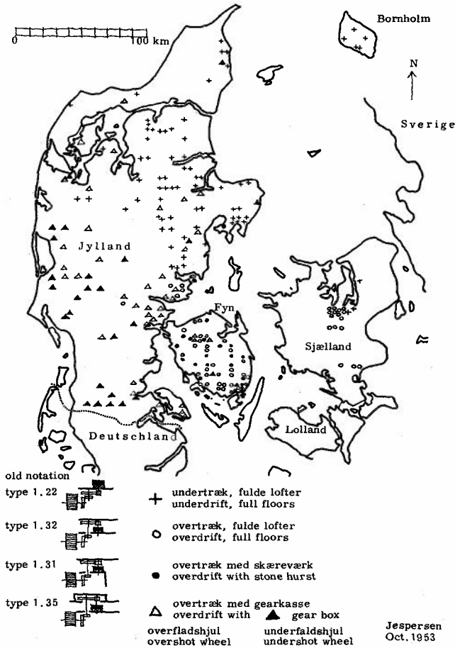
Fordeling af gangtøjstyper med stjernehjul på danske vandmøller fra 1750 til 1850.
