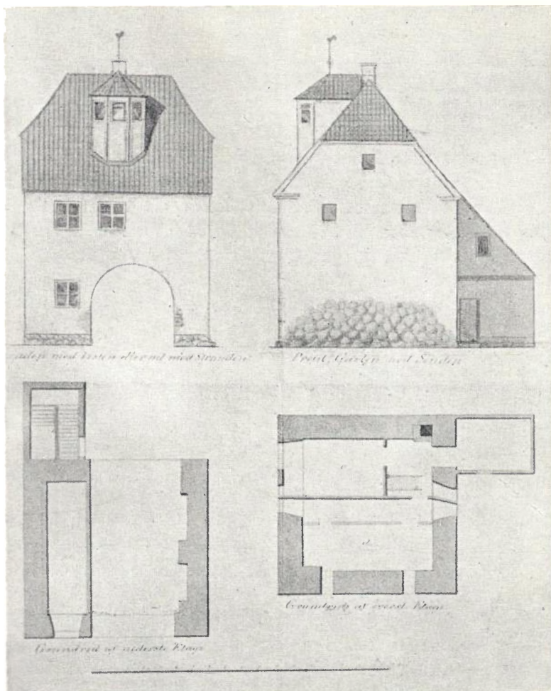
Strandporten — Facade mod Stranden; Profil af Gavlen mod Syd; Grundrids af nederste Etage; Grundrids af øverste Etage.
