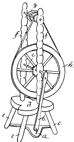
Arkitekt H. Zangenberg: Rok til at sætte i en Flaske, a) Traadlad, b) Skalen, c) Akselen, d) Skamlen, e) Ben, f) Opstandere, g) Ten, h) Hjul.
