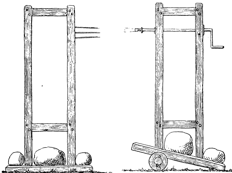
Arkitekt H. Zangenberg: Redskaber til Rebslagning.
