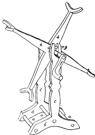
Arkitekt H. Zangenberg: Garnvinde (Haspe) til at sætte i en Flaske, a) Tværpind, b) Fodstykker, c) Opstandere, e) Aksel, f) Haandstag og Sving, g) Pind over Akselen, h) Vingerne.
