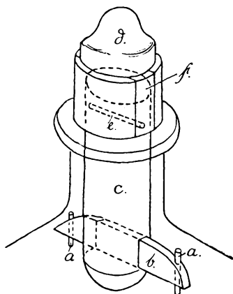
Arkitekt H. Zangenberg: Told til en Flaske med Rok eller Garnvinde (Haspe), a) Tværpind i Splitten, b) Splitten, c) Tolden, d) Hovedet til Tolden, e) Tværpind, der holder Told og Hoved sammen, f) smaa Skodder, der dækker Tværpindens Ender.
