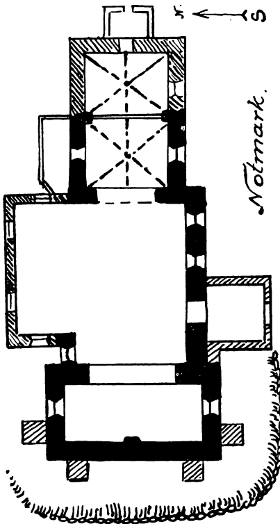
Grundrids af Notmark Kirke. Det sorte viser de fra Middel- alderen bevarede Mure. Det skrave- rede er senere Tilbygninger.
