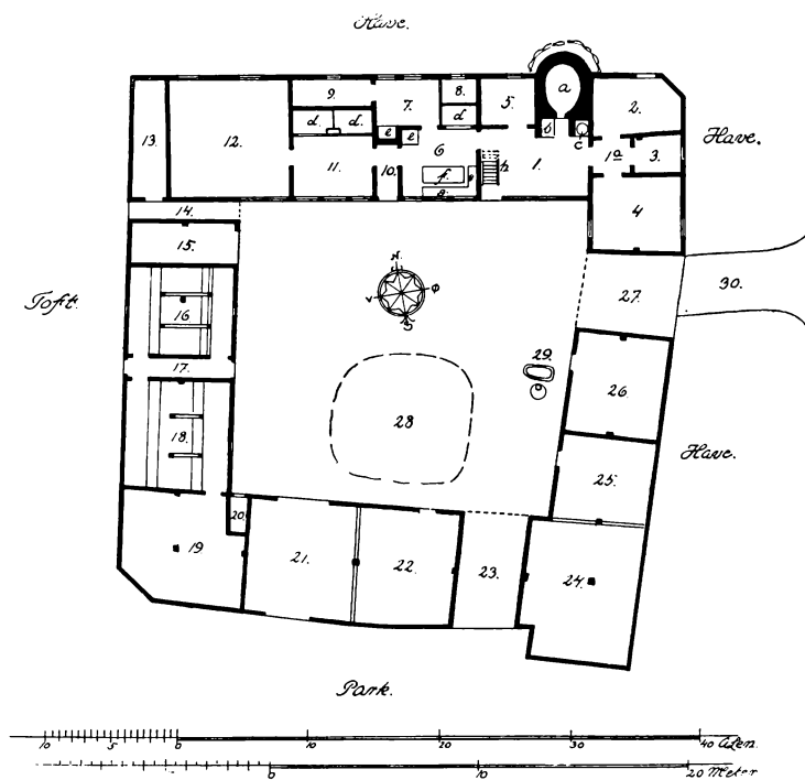
Fig. 5. Grundplan af en Gaard i Skaarup, Dreslette Sogn.
