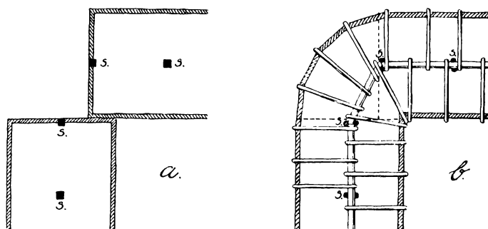
Fig. 7. Sammenbygning af to Sulelænger med et rundt Hjørne paa en Gaard i Katterød, Diernæs Sogn.
