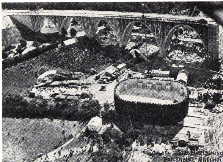
En sænkekasse til den 1. Lillebæltsbro skal løbe af stabelen, og tusinder er strømmet til
