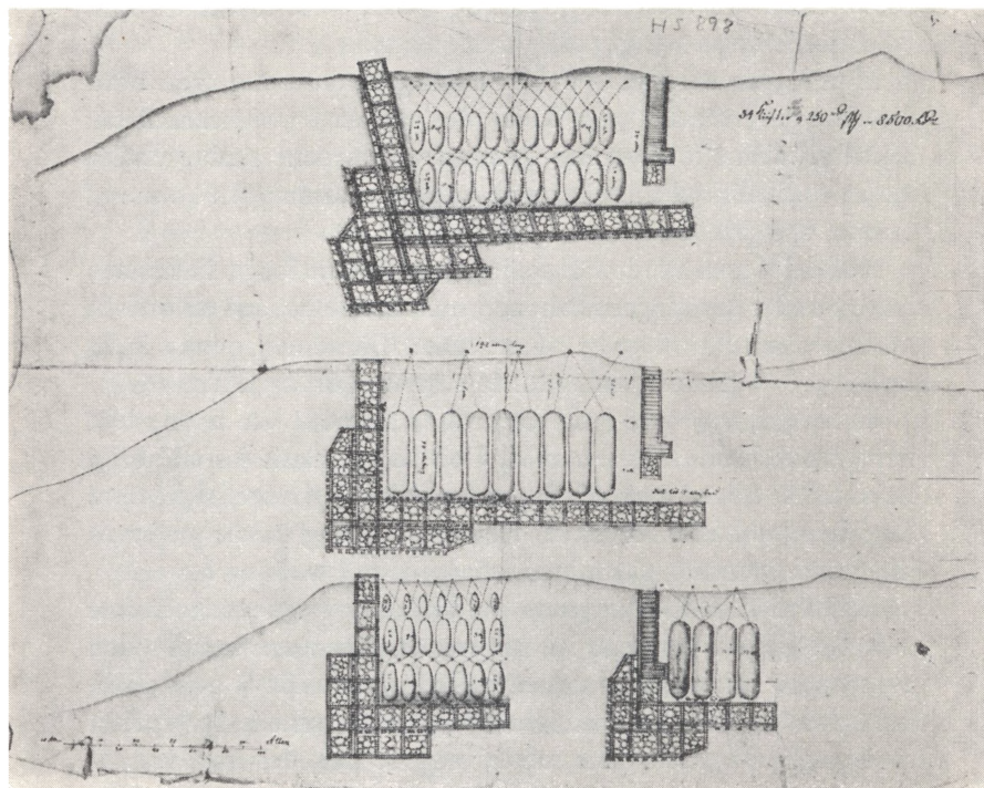
Fig. 6. Skitseprojekter til en havn syd for Helsingør ud for Svingelen, udført som led i diskussionen om Claessens havneplaner. – RA. Orlogsværftets Aflevering 1945, Designation D.
