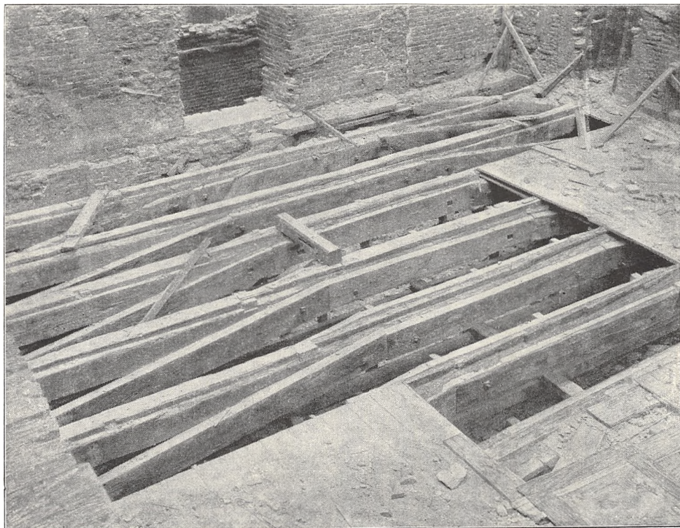
Sprængværk under Drabantsalen. Fot.
