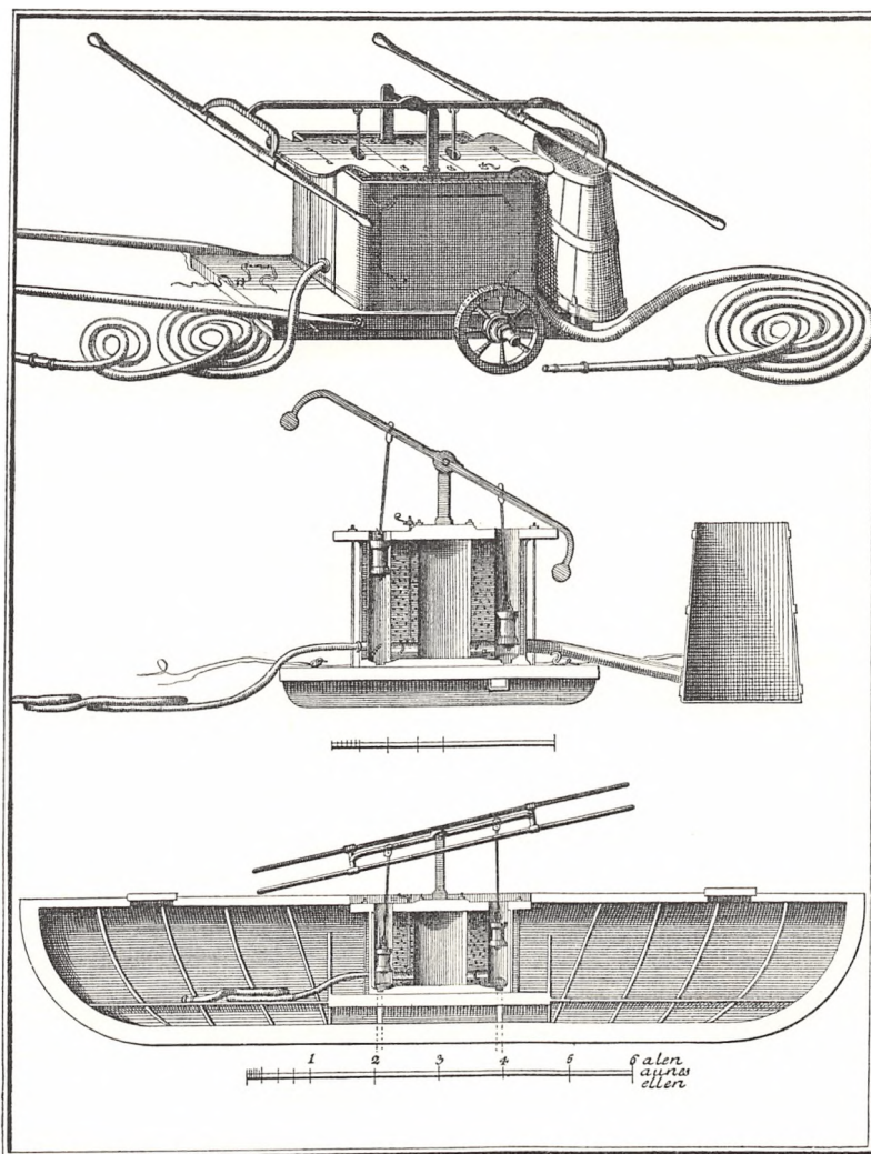
En af de store Sprøjter (foroven) og en Pramsprøjte. Thurah: Hafnia hodierna, 1748, Pl. II.
