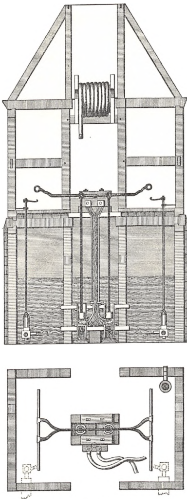
Trykværket ved Nikolaj Kirke. Thurah: Hafnia hodierna, 1748, Pl. III.
