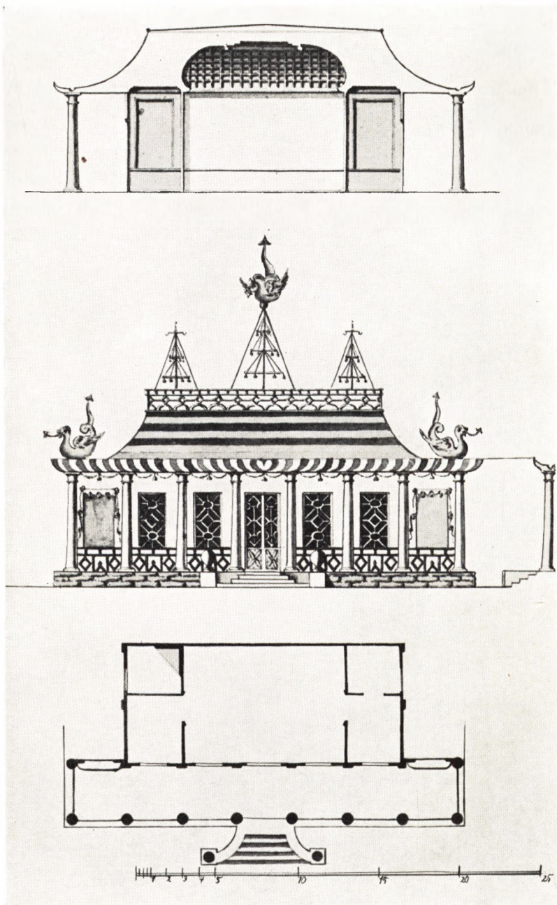
DEN FØRST APPROBEREDE PLAN TIL KINESISKE LYSTHUS. Tegning i Rigsarkivet.
