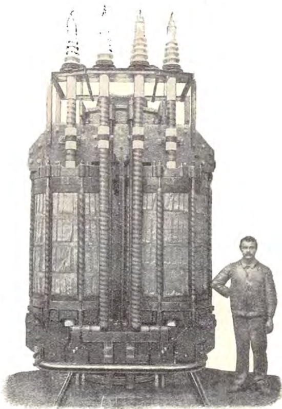
En Spændingsomformer eller Transformator for 2500 Hestekræfter og 60,000 Volts Højspænding.
