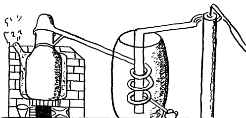
Fig. II. Brænderiapparat med spiralerør, efter J. With: Anvisning til at få meget og godt brændevin . . . , 1802.
