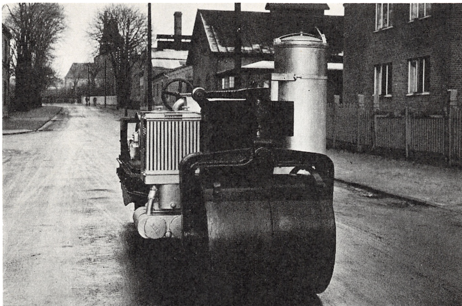
En vejtrømler (model fra slutningen af 1930'erne) påmonteret gengasanlæg. Billedet er fra Ringsted Jernstøberi & Maskinfabriks arkiv. Det viser, hvorledes fabrikkens produkter som så meget andet kørende materiel også lod sig anvende under 2. verdenskrigs knaphed på motorbrændstof.
