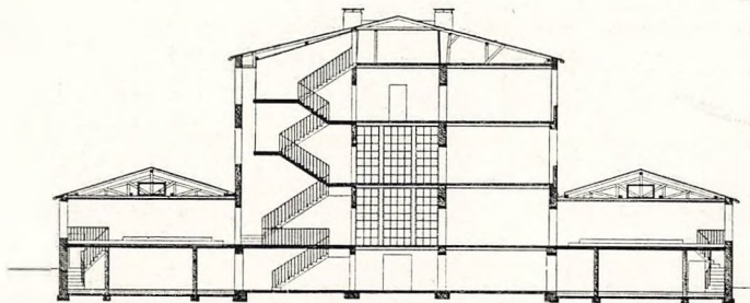
TVÆRS NIT
