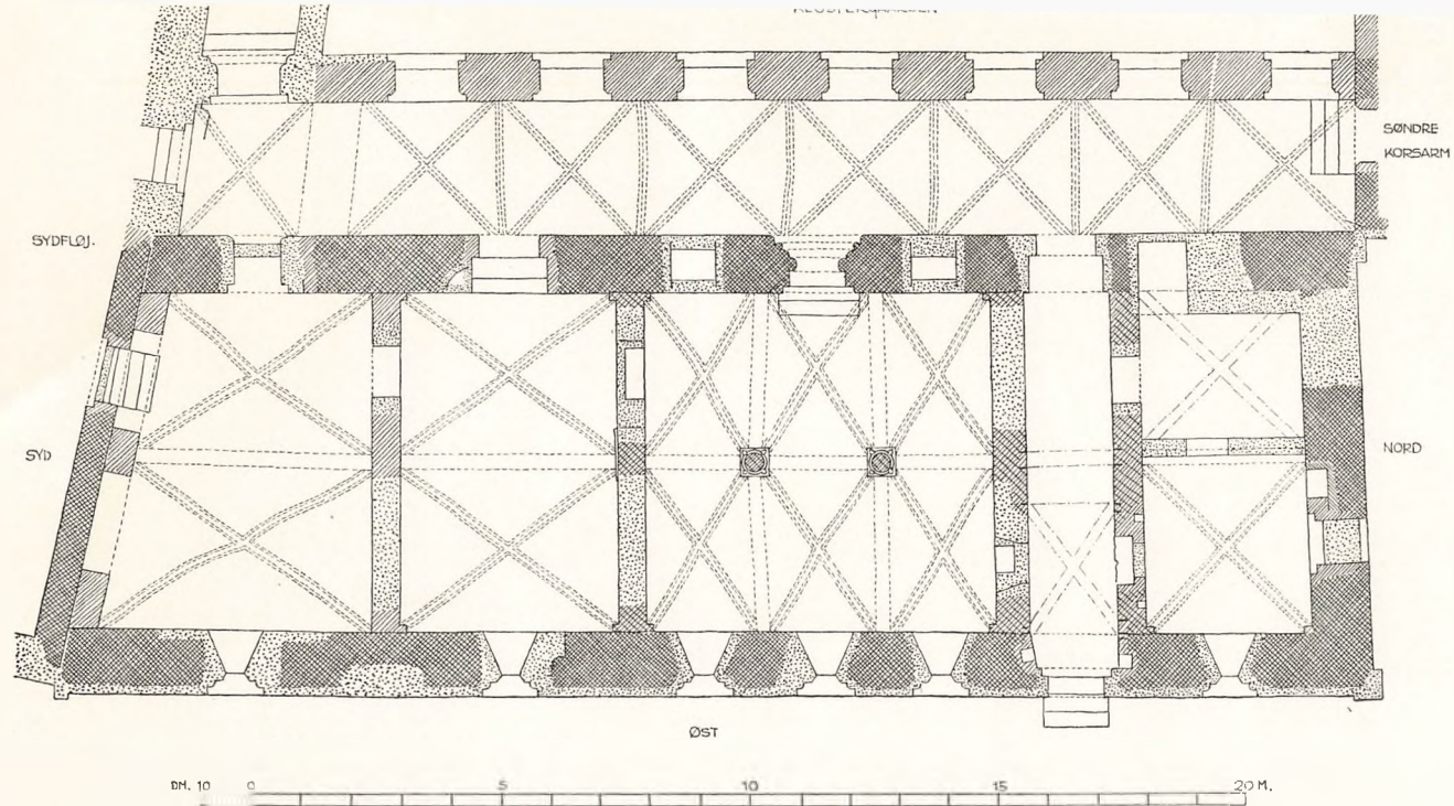
Fig. 1. Plan af Skovklosters Østfløj. Mørk Krydsskravering: oprindelig Murværk. Aaben Krydsskravering: romansk Tilbygning. Enkel Skravering: gotisk Murværk. Prikning: moderne Murværk. Rekonstrueret Hvælv og Murflugter indtegnet med stiptet Linje. Maalt af Arne Nystrøm.
