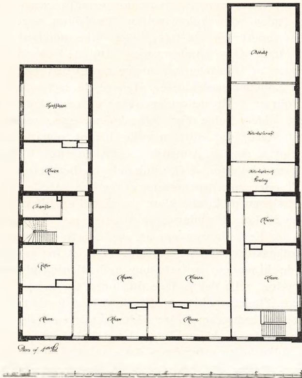
Grundplan af hovedbygningen efter 1910, 1. sal.
