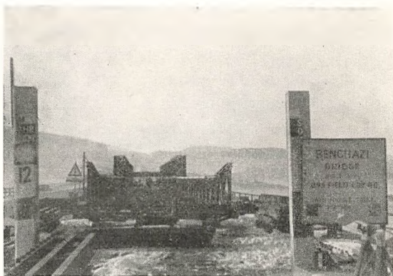
En interimistisk Bro.
