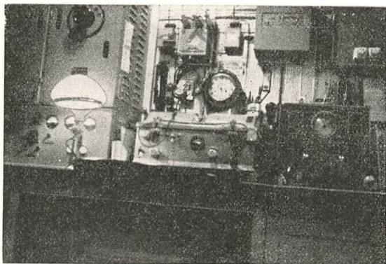
Interiør med Radiostation med Sender tv., 2 Modtagere i Midten og th. Ovenover Ladetavler og Antenneomskifter.
