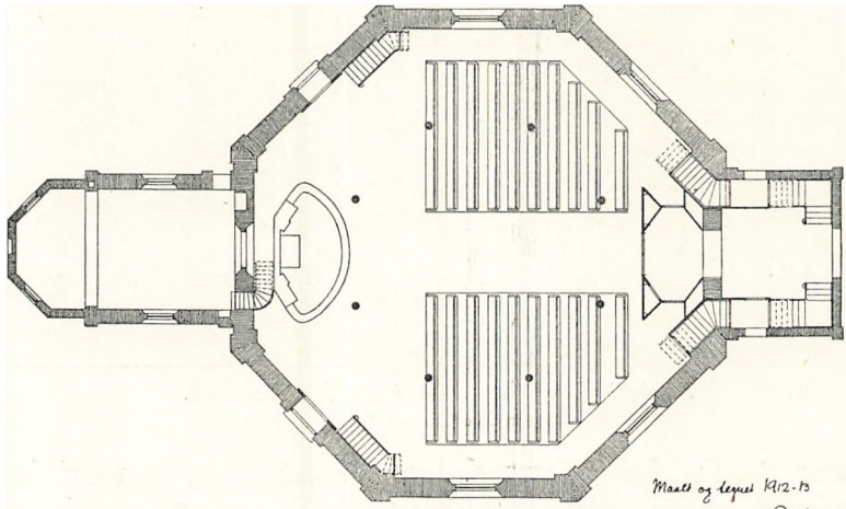
PLAN AF GULVET.
