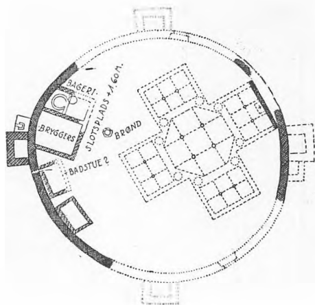
GRUNDRIDS AF ABSALONS BORG Efter Ramsing: »Kbhvns. Hist. og Topografi.« Fot. St. kgl. Bibliotek.
