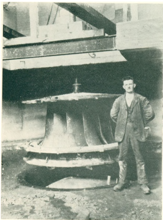
Turbine Nr. 2 bygges i den nordre Side af Aaløbet.
