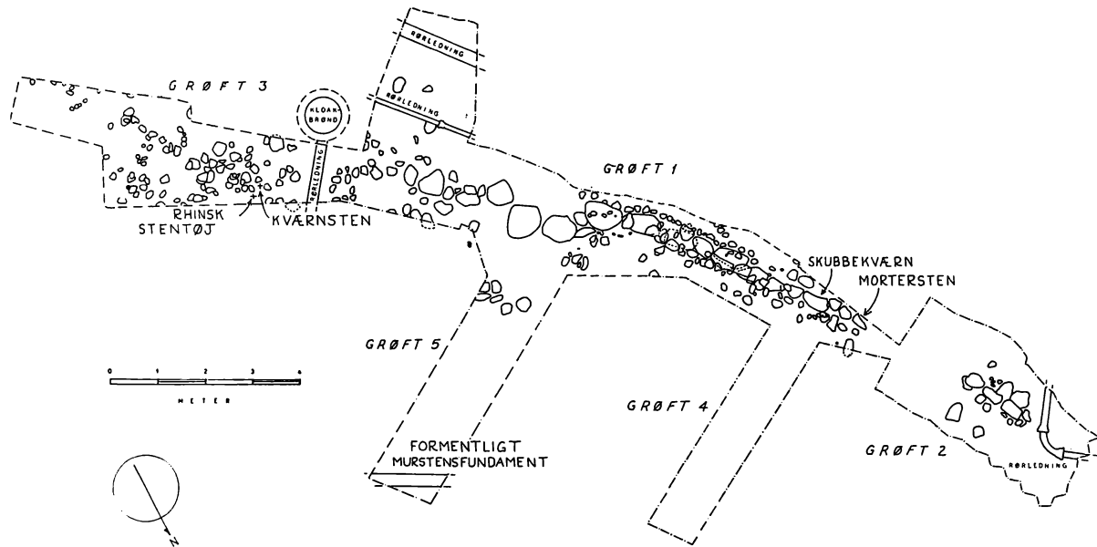
Fig. 1. Plan over udgravningen.
