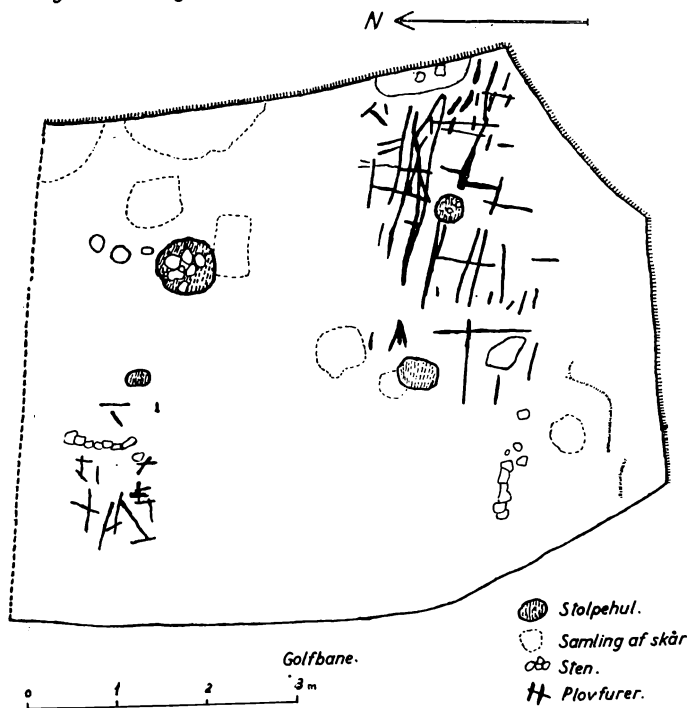
Fig. 2. Plan over den udgravede del af hustomten, med de under gulvlaget fundne pløjesor.
