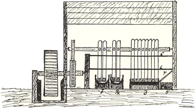
Fig. 1. Skitsen af Stampemøllen forestiller et Tværnsnit gennem Huset og Stamperiet.
