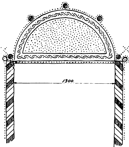
Fig. 12. Norddør. (Rekonstruktion).
