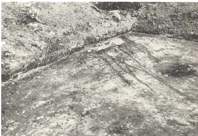
Fig. 3. Pløjesporene i det gråhvide blegsand. Tilhøjre et stolpehul med forkullede stolperester.
