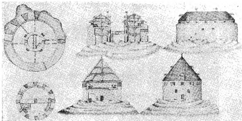
Fig. 5. Tegning af »Stortårn« foroven og »Lilletårn« forneden visende grundplan, lodret snit og tårnens ydre (Kgl. Bibliotek).
