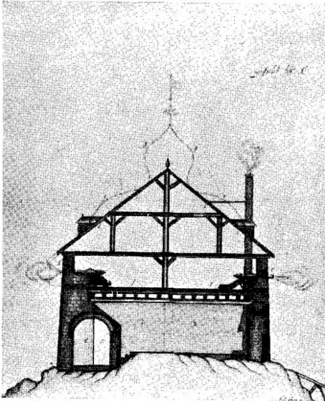
Fig. 11. Coucherons projekt til Lilletårn med krudtkammer til venstre og kamin til højre. (Rigsarkivet)
