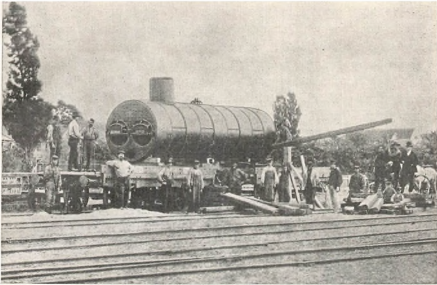
Arbejdere fra Møller & Jochumsens Fabrik i Horsens lægger en Kedel paa en Jernbanevogn, 1875. Femte Person fra venstre, Manden nederfor Fyrhullerne, er Chr. Johansen.
