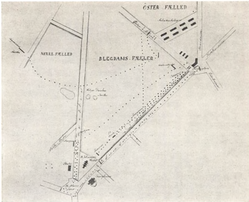
Politiets Kort til Rapport over »Fælledslaget«s Begivenheder. Husar-Afdelingerne er angivet med de sorte Streger ved Navnene Castenskjold, Moltke og Neergaard; Prikkerne disses Bevægelser. Langs Blegdamsvej angiver en Del Navne Politi-Afdelingerne under hver sin Politiasistent eller -inspektør. (Originalen i Højesterets Arkiv).
