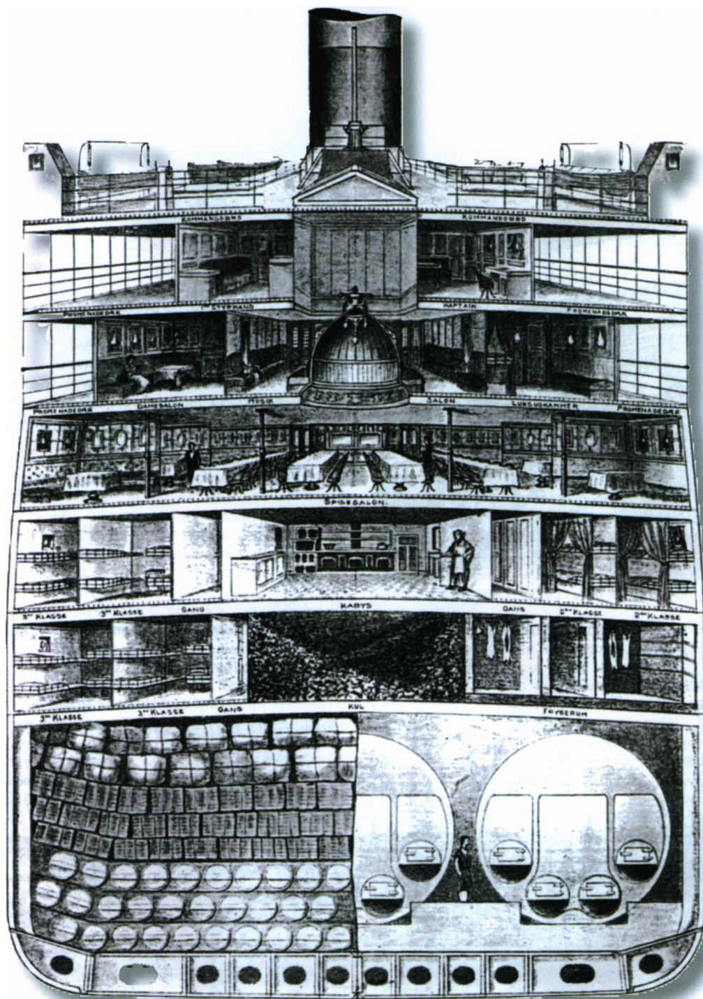
Den dobbeltskruede OSCAR II havde 6 dæk.
