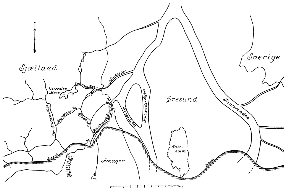
Fig. 1. Københavnsegnens Smeltevandsfloder.
