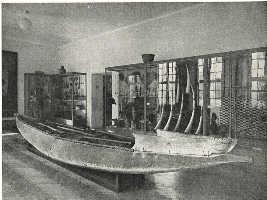
Kano hjemsendt fra de danske Kolonier paa Guineakysten. Nationalmuseet. Baaden er ca. 6,80 m lang, men har oprindeligt haft en Længde af ca. 10 m. Midterstykket er af Pladshensyn fjernet inden Sø-Transporten hjem. Der findes ikke Søm eller Nagler af nogen Art i Baaden. Alle Sammenføjninger er surrede med Plantetrevler.
