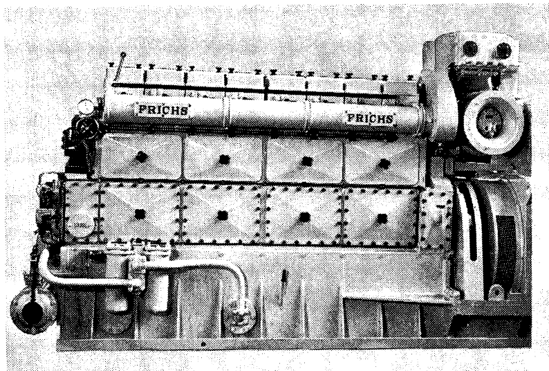
500 hk hjælpemotor type 8185 CUT med trykladning og ladeluftkøling
