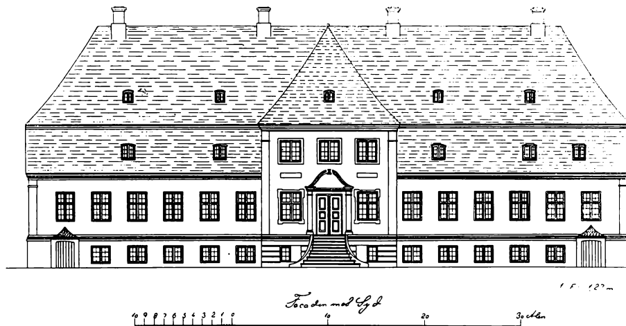
Constantinsborg. Sydfacaden efter tegning af C. Steinbrenner fra 1867.
