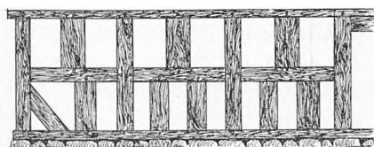
Facadeudsnit af Sydøstjysk bindingsværk.
