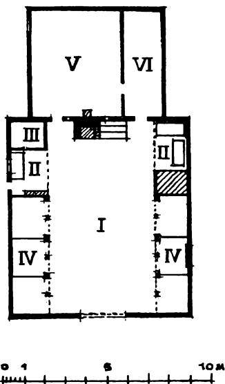
Saksisk hus fra Lille Dannevirke (efter Mejborg). I. diele, II. »de Sitten«—sidde- og sovepladser, III. kammer, IV. stalde, V. og VI. stuer.
