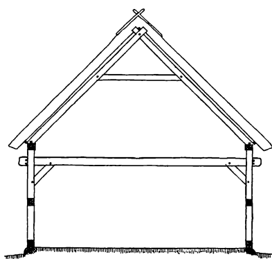
Snit af ost dansk bindingsværkshus.
