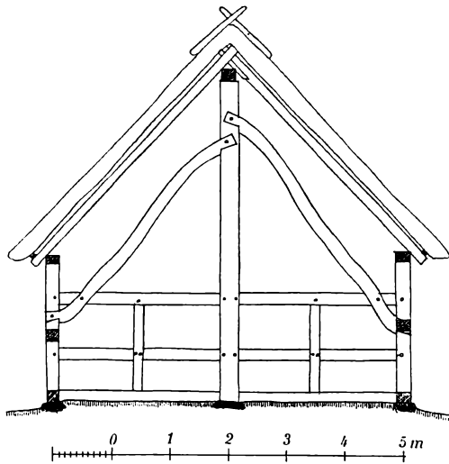
Snit af vestfynsk sulehus af ældste form.
