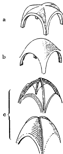
a. Romansk krydshvælv. — b. Senromansk kuppelagtigt hvælv. — c. Gotisk krydshvælv.
