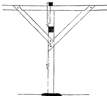
Længdeudsnit, visende højremsstolpe med skråbånd.
