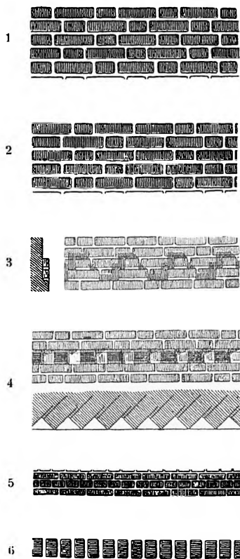
1. polsk skifte, 2. munkeskifte, 3. bloktandsgesims, 4. savskifte, 5. blokskifte, 6. rulskifte.
